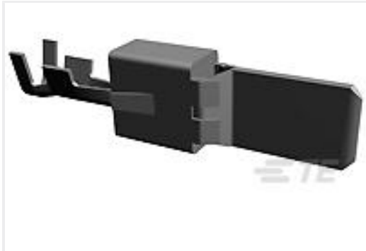
TE Part #963766-2 TAB 9.5x1.2 CONTACT CF SRC Sn
