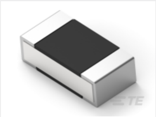
TE Part #2176306-6 RP 1E 0.1W 1K3 0.1% 25PPM 5K RL
