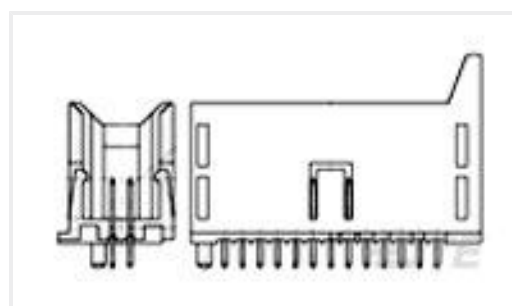
TE Part #827881-3 2X13P MOD2 ST-STECK
