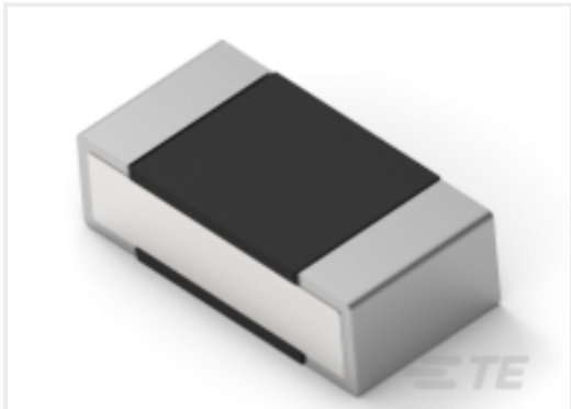
TE Part #2176312-2 RP 1E 0.1W 12K7 0.1% 25PPM 1K RL
