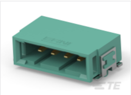
TE Part #384473-E SRCA 2,54 4 M 1 SMD 137 E1 167 * GURT *
