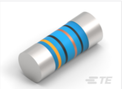
TE Part #2176316-6 MELF SMA_A 270R 0.1% 15PPM 0207 1W
