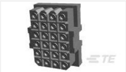
TE Part #207532-9 SKT HDR ASSY,24 POSN,METRIMATE
